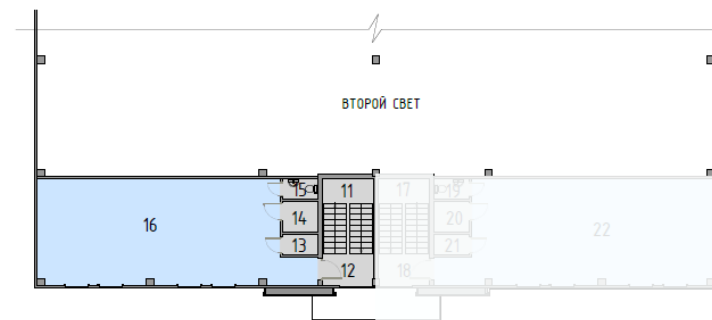
План 2 этажа
