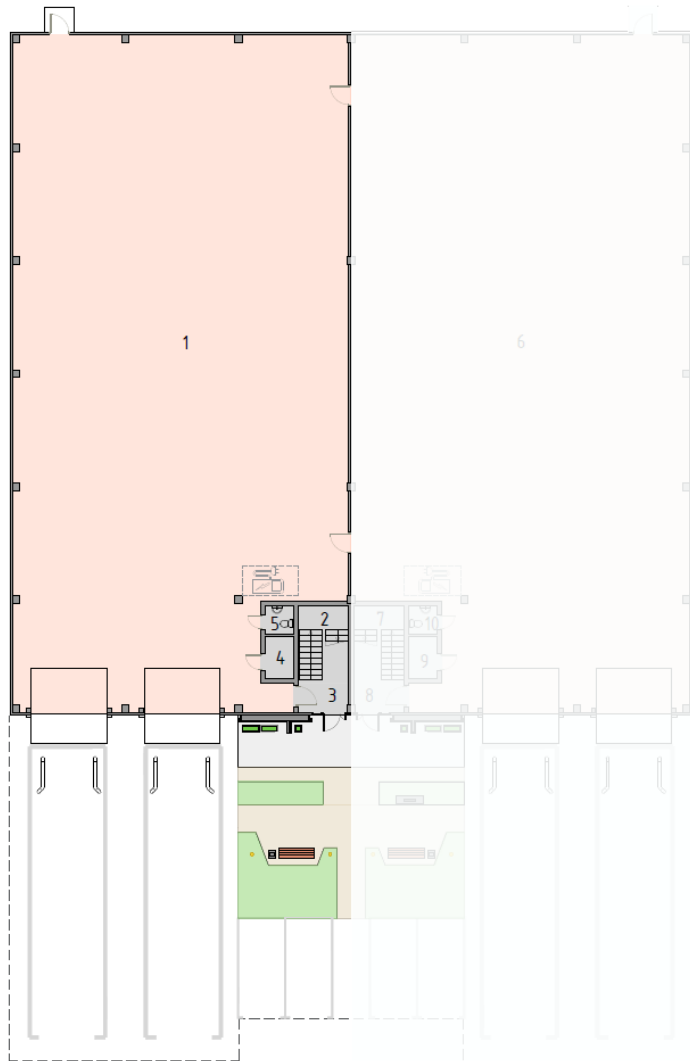
План 1 этажа
